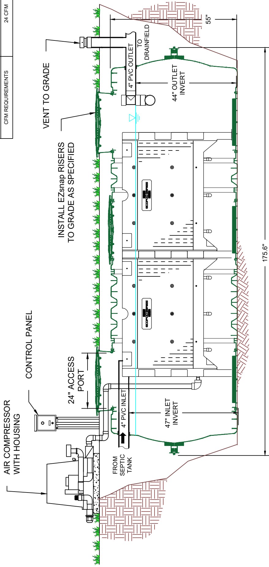
E100-N IM-1530 REACTOR TANK
